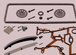
febi 33082 pentru: Opel, Vauxhall (benzină) Urmați instrucțiunile de asamblare.
