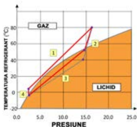
Fig. 1. Circuitul ilustrativ al agentului refrigerant R134a în sistemul de aer condiționat auto.
